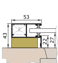
Termikusan leválasztott K53VT vezetősín
