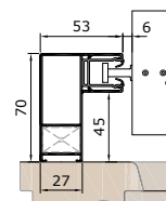
ED53V vezetősín
