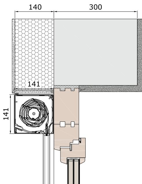
Hőszigetelés és tokmagasítással. VORO SE.
