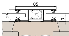
K85V vezetősín
