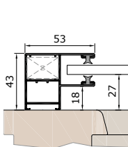
KA53V vezetősín
