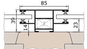
KE85V vezetősín
