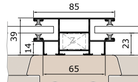
KF85V vezetősín
