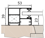
KF53V vezetősín
