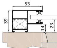
KE53V vezetősín felújításhoz
