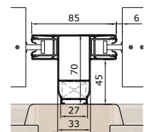
ED85V vezetősín
