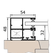
KR54V vezetősín
