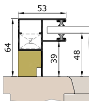
Termikusan leválasztott K53VT vezetősín
