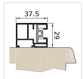
Z37V vezetősín
