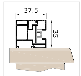
FS Z37VP vezetősín, vakolt módzat
