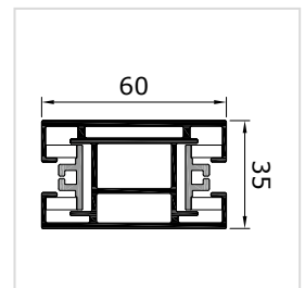
Önhordó ikersín FS ZT60V
