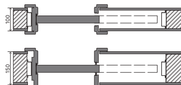
KOMPACT ÁTJÁRÓ TOKOK 100 ÉS 150 MM FALVASTAGSÁGOKHOZ
