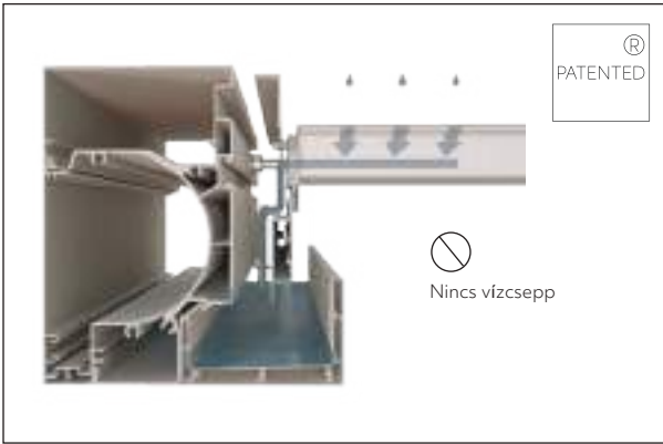
Vízvezető rendszer
