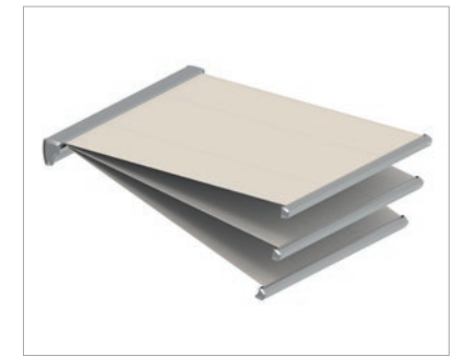
A VIVA 7040 napellenző dőlésszöge opcionálisan motorral (Variotronic) vagy tekerőkarral (Variomatic) állítható.
