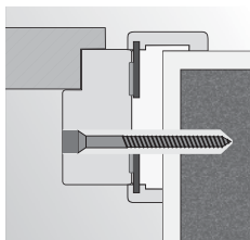
Beépítés purhabbal és dűbellel kőműves falba
