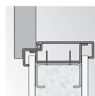
nagy saroktokok beépítése gipszkarton falba
