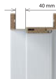
maximum ajtótok szélesebb tollal lehetőség felárért
