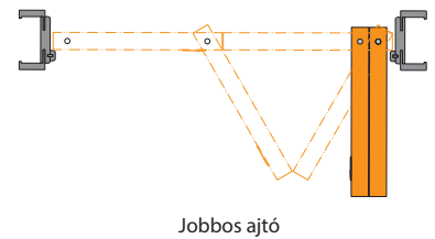
AJTÓNYITÁSI MÓDSZER* (felülnézet)
