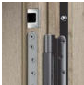
4 betörésbiztos kiemelésgátló csap professzionális pánttal (II. típus)
