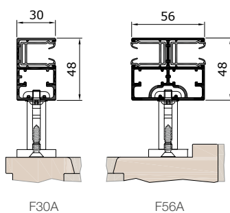
Vezetősinék RAFF A
