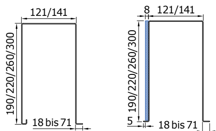
Nyílásnagyságok RAFF F
