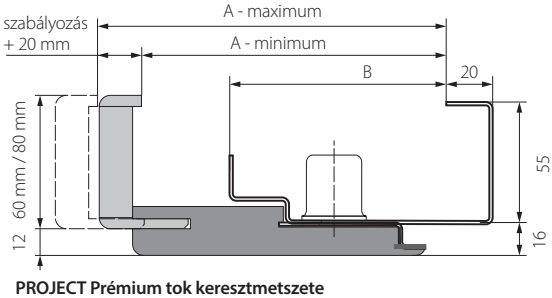
PROJECT Prémium tok keresztmetszete
