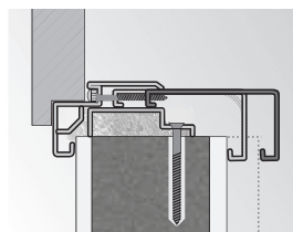
Állítható tok
