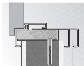
Állítható tok "sarkos éllel"
