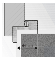
KIS saroktok
